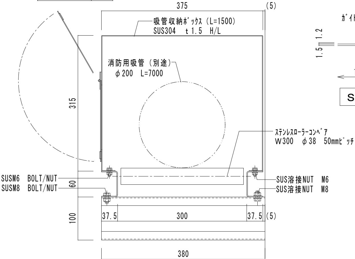
正面図 (S=1/5)
