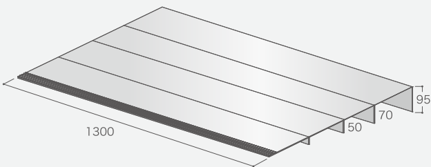
キヨレックススロープ H50、H70、H95 (勾配 1/8)
