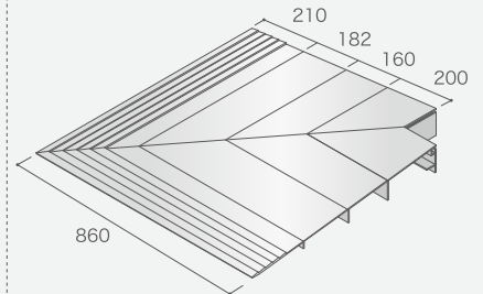
キヨレックススロープ出隅 H50、H70、H95
