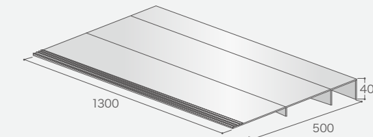
キヨレックススロープH40 ロングタイプ (勾配 1/12.5)
