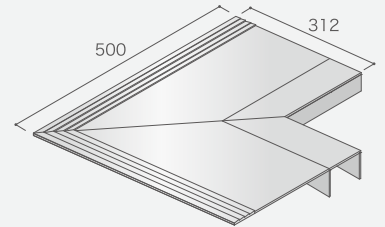
キヨレックススロープ出隅 H40
