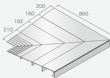
キヨレックススロープ入隅 H50、H70、H95
