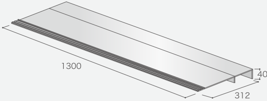
キヨレックススロープ H40 (勾配 1/8)
