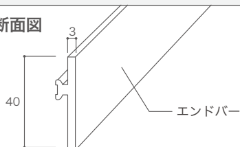
キヨレックススロープH40 ロングタイプ (勾配 1/12.5)
